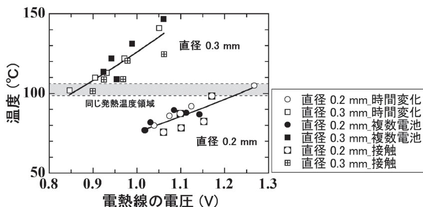
図5 長さ50 mm直径0.2 mm、0.3 mmの電熱線にかかる電圧と発熱温度の関係。時間変化（○、□）に関しては電圧の大きい方からそれぞれ0、0.5、1、2、4時間後の測定値である（なお、直径0.2 mmの4時間後の実測値は他のマーカーと重なっており見えないが電圧1.02 V、温度77℃である）。他の測定値は測定順番と測定値の変化に相関はなく、電熱線に乾電池をつないでから50～180秒間の電熱線にかかる電圧と温度の平均値それぞれ5点を示した。また、破線で囲まれた領域は直径が異なる電熱線にも関わらず、発熱温度領域が重なる範囲を意味する。
