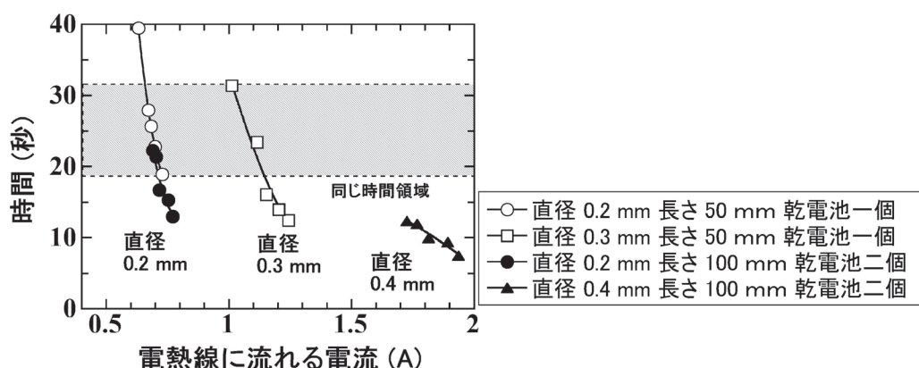
図8 乾電池を使用した長さ50 mm（直径0.2 mmと0.3 mm）、長さ100 mm（直径0.2 mmと0.4 mm）の電熱線に流れる電流と発泡ポリスチレンを溶かす時間の関係。
