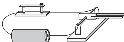
図1 「電気による発熱」実験外観図。乾電池は単1のアルカリ電池を使用した。
