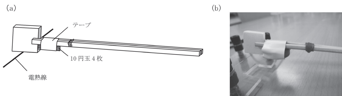
図7 (a)発泡ポリスチレンを溶かす場面の概略図と(b)実物写真。
