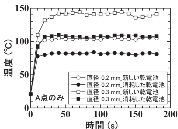
図4 長さ50 mm直径0.2 mm、0.3 mmの電熱線の電源投入後の温度変化。新品の乾電池に関する値は図3(a)と同様のものを採用した。
