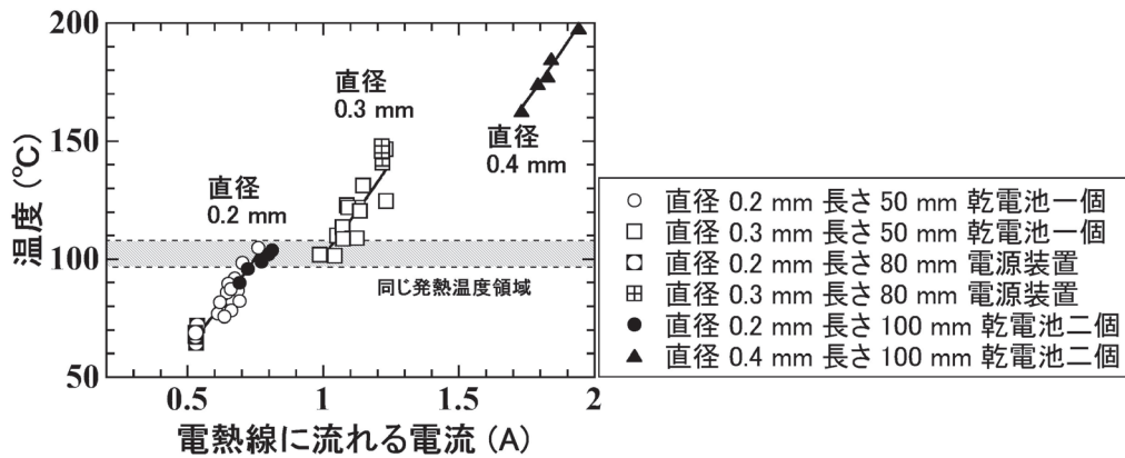
図6 (a図) 直径0.2 mm、長さ50 mm及び100 mmの電熱線にかかる電圧と発熱温度の関係。(b図) 電熱線に流れる電流と発熱温度の関係。直径0.2 mmにおける文献値を破線で示した。(c図) 乾電池を使用した長さ50 mm (直径0.2 mmと0.3 mm) と長さ100 mm (直径0.2 mmと0.4 mm)、および電源装置 (乾電池1個相当) を使用した長さ80 mm (直径0.2 mmと0.3 mm) の電熱線に流れる電流と発熱温度の関係。なお、長さ50 mmの結果は前章で測定したデータであり、長さ100 mmおよび電源装置を使用した長さ80 mmの結果については、使用済み乾電池を無作為に選び、配線には十分配慮し5回測定したものである。電源装置は、ヤガミ製DS-9 V(新型：新教育課程用に製造・販売された物)を使用した。
