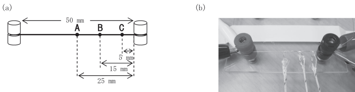
図2 (a) 熱電対の取り付け位置の概略図と (b) 実物写真。
