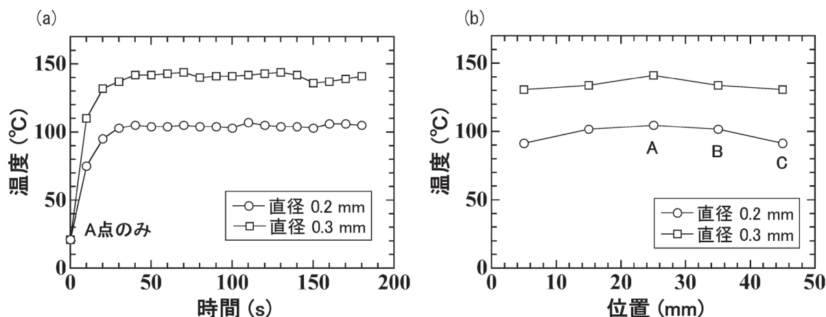
図3 長さ50 mm電熱線の中央部(A点)における電源投入後の温度変化((a)図)及び安定後の電熱線の温度分布((b)図)。(a)図において電熱線の温度が安定したと考えた測定開始後50秒から180秒までの温度と電熱線にかかる電圧の平均値は、直径0.2 mmにおいてはそれぞれ104.6°Cと1.27 V、直径0.3 mmにおいてはそれぞれ141.1°Cと1.05 Vであった。
