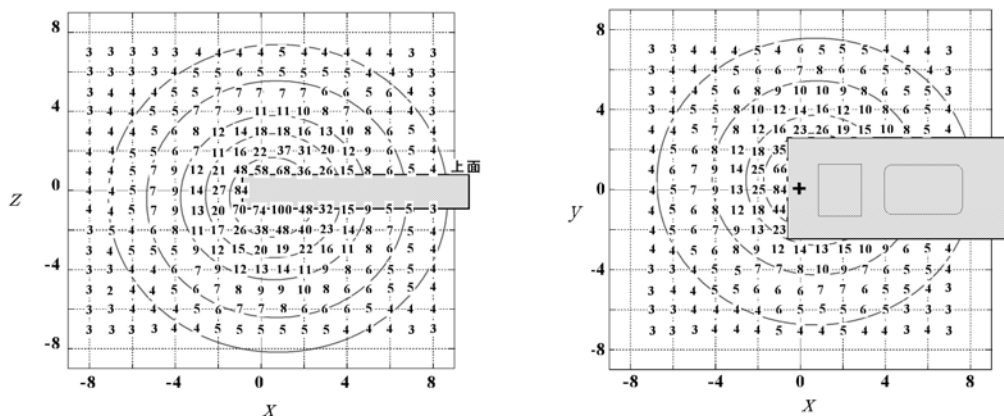
図7 「はかるくんⅡ」測定分布。(左)xz面、(右)xy面。最大値 4.632 \mu\text{Sv/h} を100として百分率で表している。
