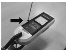
図3 測定の様子。棒の先(矢印)の線源を移動させて測定を行った。
