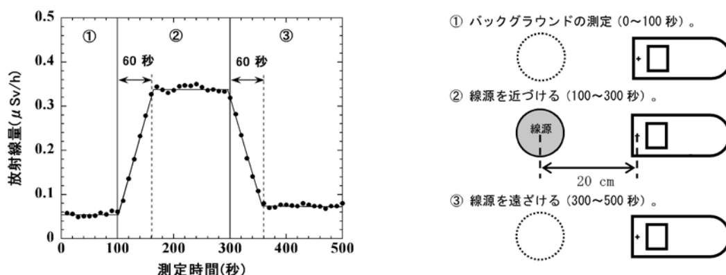
図8 (左)「はかるくん」の測定値の時間変化。10秒ごとの測定を500秒間行った。安定した時間の平均値は、①0～100秒： 0.056 \mu\text{Sv/h} 、②160～300秒： 0.338 \mu\text{Sv/h} 、③360～500秒： 0.075 \mu\text{Sv/h} であった。(右)実験方法の概略図。なお、「はかるくん」と線源の距離は、+印から線源の中心まで20cmである。
