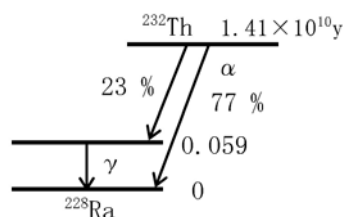
図4 ^{232}\text{Th} の崩壊図 11) 。エネルギーの違う2本の \alpha 線と、 \gamma 線を出している。
