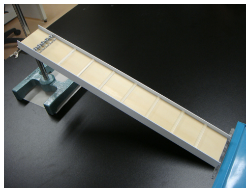
図 5. 洗濯板モデルの外観図(a)と実物写真(b)。傾斜の変化は実験用スタンドを用いた。
