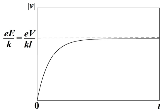
図 2. (8)式による電子の速度の時間変化。時間の経過とともに一定速度に近づく。
